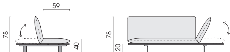
Seitenansicht Metallfuß
