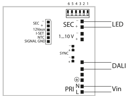
DALI diagram - Collegamento DALI
